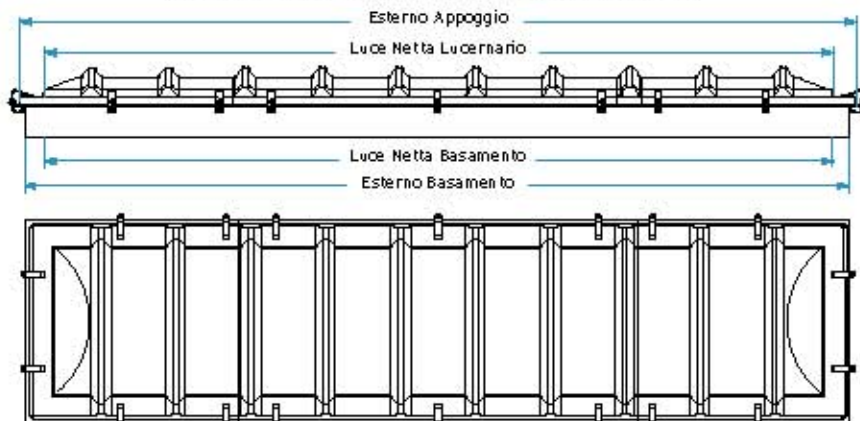
SEZIONE LUCERNARIO REALIZZATO IN PC ALV
