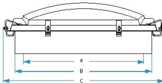
SEZIONE LUCERNARIO REALIZZATO IN PC O PMMA
